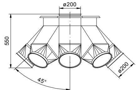
Drehrundverteiler 8 - fach 45° Ø200 Art. Nr.: 106945
