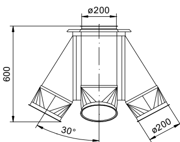
Drehrundverteiler 4 - fach 60° Ø200 Art. Nr.: 106939
