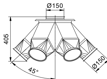
Drehrundverteiler 6 - fach 45° Ø150 Art. Nr.: 106743
