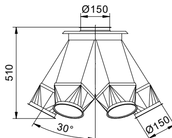
Drehrundverteiler 6 - fach 60° Ø150 Art. Nr.: 106754
