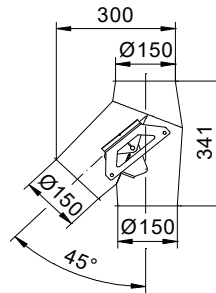
Zweiwegeverteiler 1x45° verzinkt Ø150 Art. Nr.: 106816
