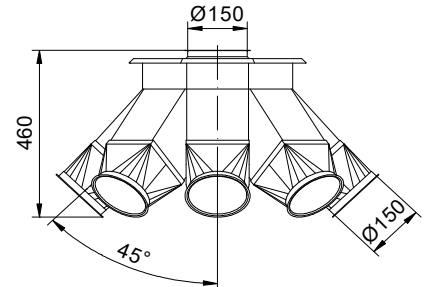
Drehrundverteiler 8 - fach 45° Ø150 Art. Nr.: 106767
