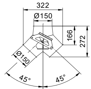
Drehrundverteiler 8 - fach 45° Ø150 Art. Nr.: 106767
