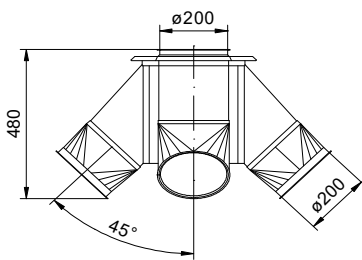
Drehrundverteiler 4 - fach 45° Ø200 Art. Nr.: 106937
