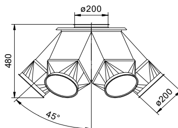
Drehrundverteiler 6 - fach 45° Ø200 Art. Nr.: 106941
