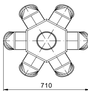
Drehrundverteiler 6 - fach 60° Ø150 Art. Nr.: 106754
