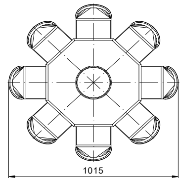
Drehrundverteiler 8 - fach 60° Ø200 Art. Nr.: 106947
