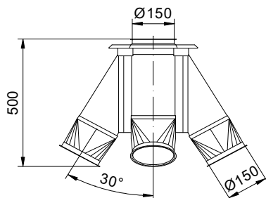
Drehrundverteiler 4 - fach 60° Ø150 Art. Nr.: 106731
