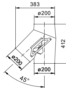
Zweiwegeverteiler 1x45° verzinkt Ø200 Art. Nr.: 106933
