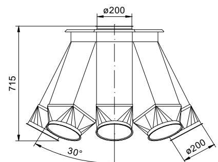
Drehrundverteiler 8 - fach 60° Ø200 Art. Nr.: 106947
