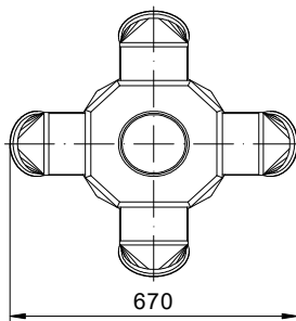
Drehrundverteiler 4 - fach 60° Ø150 Art. Nr.: 106731
