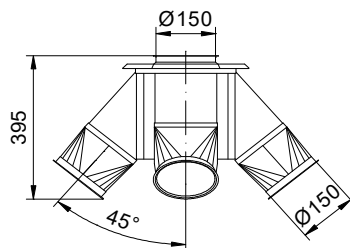
Drehrundverteiler 4 - fach 45° Ø150 Art. Nr.: 106720
