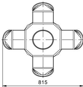
Drehrundverteiler 4 - fach 60° Ø200 Art. Nr.: 106939
