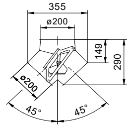
Drehrundverteiler 8 - fach 45° Ø200 Art. Nr.: 106945
