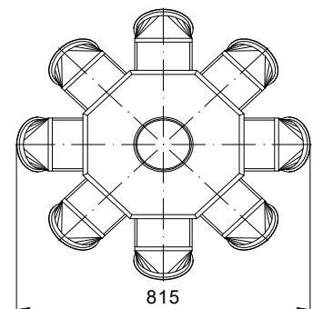
Drehrundverteiler 8 - fach 60° Ø150 Art. Nr.: 106778
