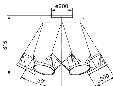
Drehrundverteiler 6 - fach 60° Ø200 Art. Nr.: 106943
