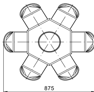
Drehrundverteiler 6 - fach 60° Ø200 Art. Nr.: 106943
