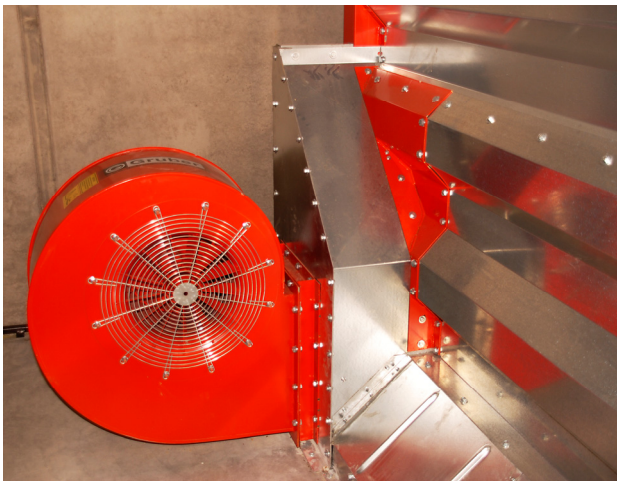
HL-Belüftungsgebläse am rückwärts innenliegenden Luftschacht angebaut
