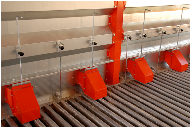
Frontsockel mit eingebauten Auslaufschiebern und Bedienungsgestänge für Luftklappen
