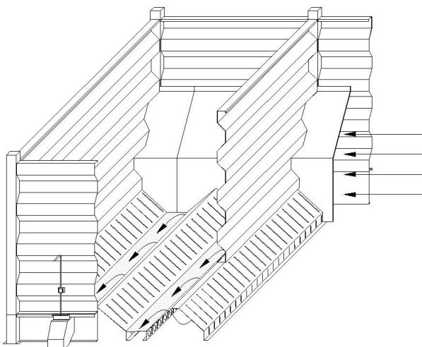
HL-Belüftungsgebläse am rückwärts innenliegenden Luftschacht angebaut
