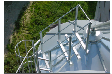
Dacheinstiegs Luke mit Dachleiter und Geländer
