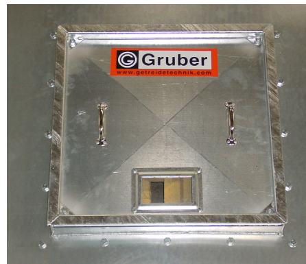
Einstiegs Luke mit Sichtfenster
