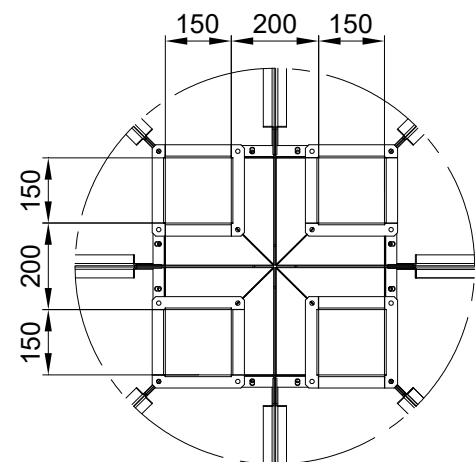
Detailskizze Auslauf
