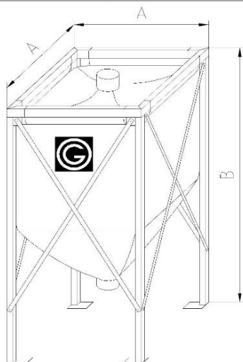
Gewebe-Silo mit Gestell
